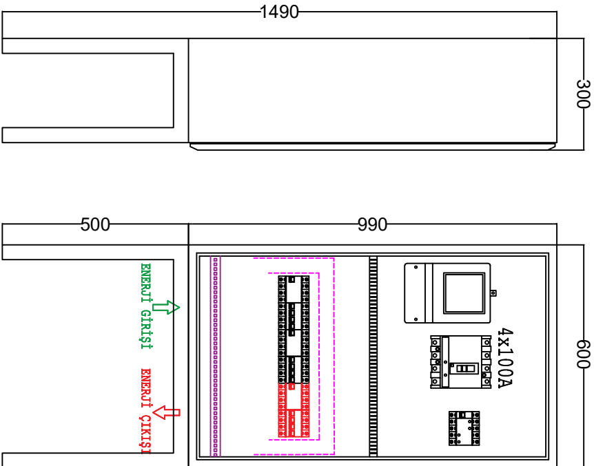
YAN GÖRÜNÜM
