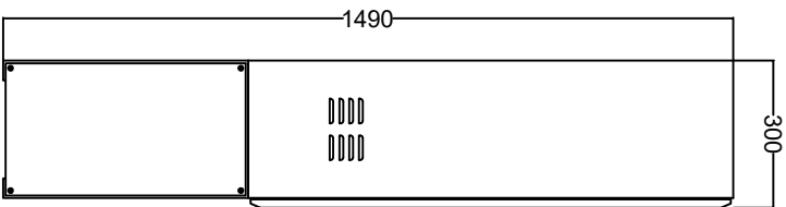
YAN GÖRÜNÜM
