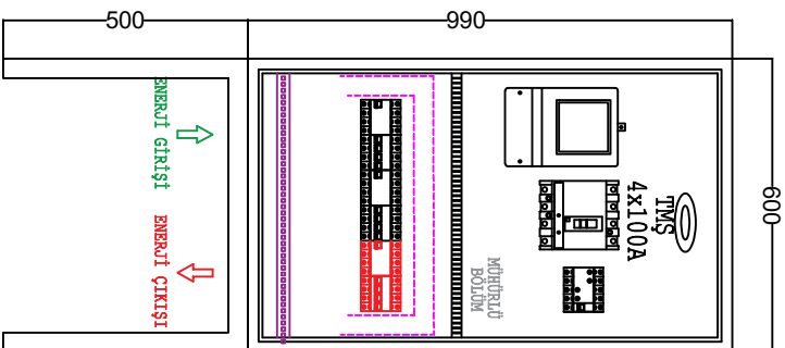
ŞALT MALZEMELİ İÇ GÖRÜNÜM
