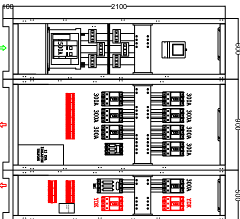
ŞALT MALZEMELİ İÇ GÖRÜNÜM
