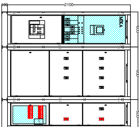
PERDE SACLI İÇ GÖRÜNÜMÜ
