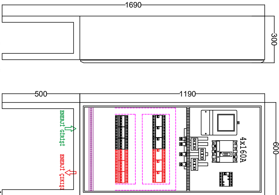
YAN GÖRÜNÜM
