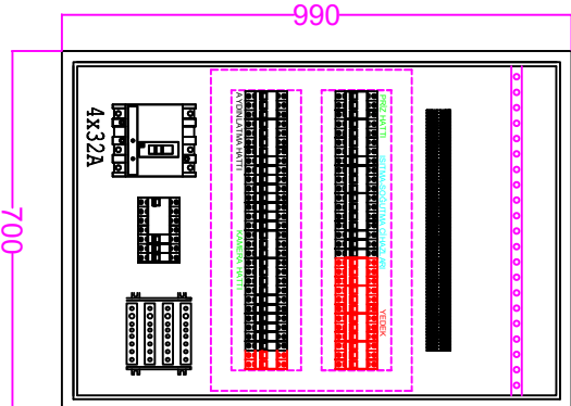
ŞALT MALZEMELİ İÇ GÖRÜNÜM
