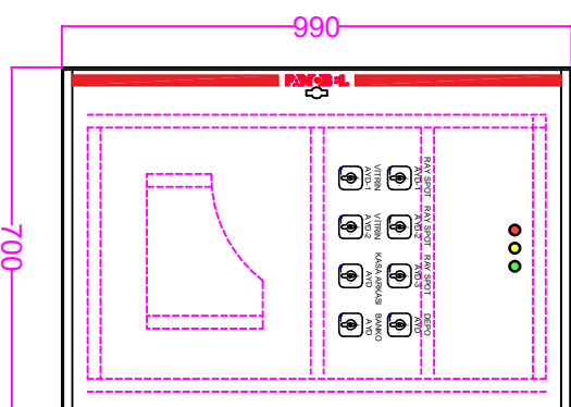
SAC KAPILI DIŞ GÖRÜNÜM
