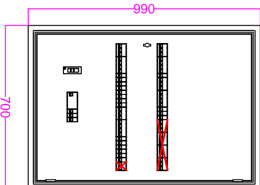
PERDE SACLI İÇ GÖRÜNÜM
