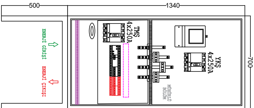
ŞALT MALZEMELİ İÇ GÖRÜNÜM
