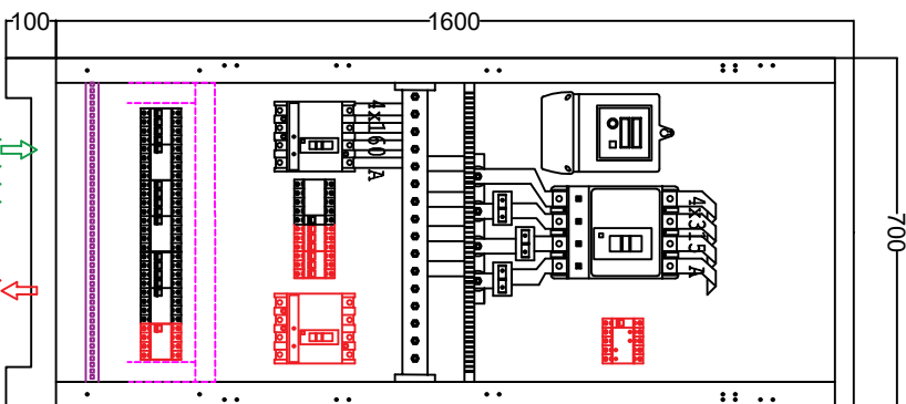
ŞALT MALZEMELİ İÇ GÖRÜNÜM
